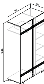
Шкаф 2-ух створчатый Ш2
