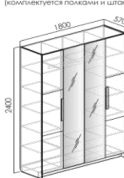
Шкаф 4-ех створчатый Ш6 с зеркальными фасадами (комплектуется полками и штангой)
