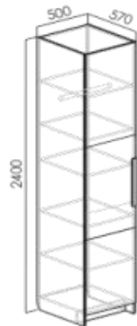
Шкаф-пенал Ш1 (комплектуется полками и штангой)
