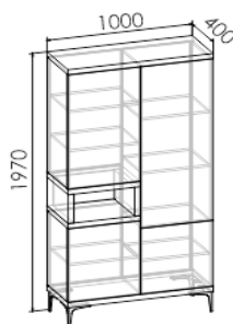
Шкаф Ш1 правый
