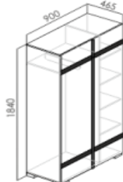
Шкаф 2-ух створчатый Ш2 (комплектуется полками и штангой)
