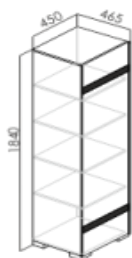
Шкаф пенал Ш1 (комплектуется полками)
