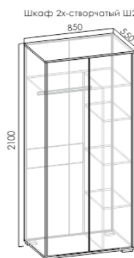
Шкаф 2х-створчатый Ш2
