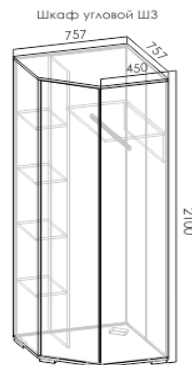
Шкаф угловой Ш3
