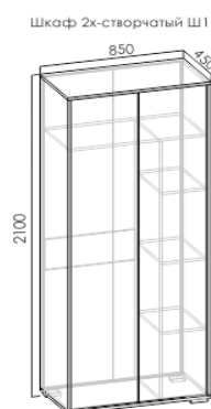
Шкаф 2х-створчатый Ш1
