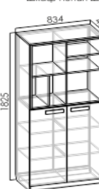
Шкаф-пенал Ш2
